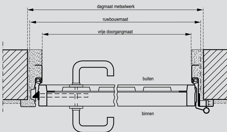
Doorsnedetekening bij binnenaanslag
