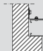
doorsnede A alternatief 2
