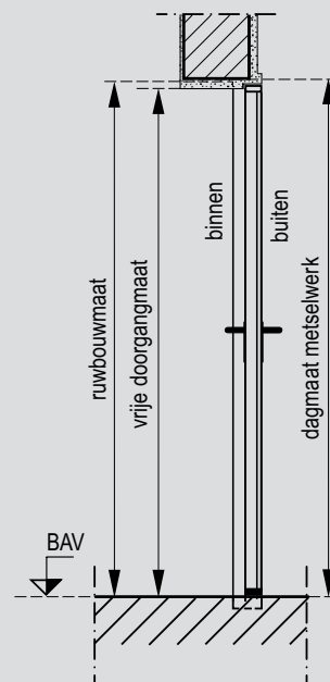
Inbouw bij buitenaanslag
