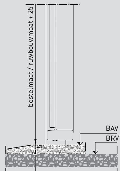
detail A : zonder aanslag
