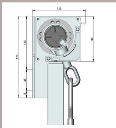
Doorsnede en maatvoering
